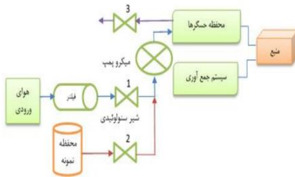
شکل ۱. نمای کلی و شماتیک سامانه بینی الکترونیک در هنگام آزمایش
