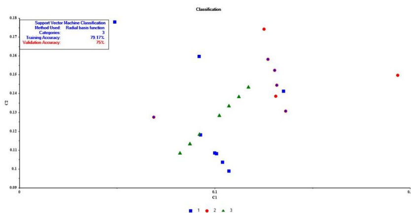
شکل ۳. نتایج SVM برای طبقه‌بندی ارقام نمونه‌های گندم
