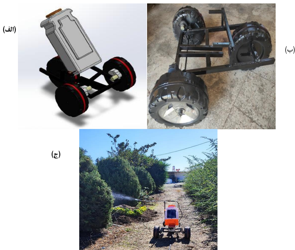
شکل ۱- (الف) طراحی ربات سمپاش در نرم‌افزار سالدورکس، (ب) شاسی و چرخ‌های ربات و (ج) ربات سمپاش خودکار خورشیدی
