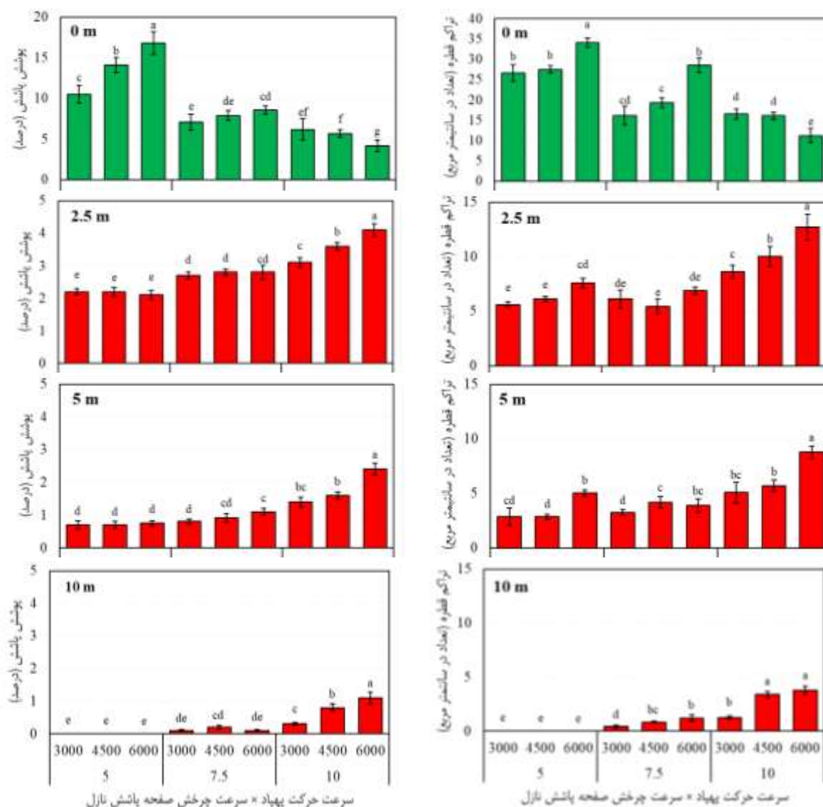
شکل ۱. اثر سرعت حرکت (۵، ۷/۵ و ۱۰ متر بر ثانیه) و سرعت چرخش نازل میکرونی (۳۰۰۰، ۴۵۰۰ و ۶۰۰۰ دور در دقیقه) پهپاد بر پوشش و تراکم قطرات پاشش در مرکز کرت (۰ متر) که مد نظر و مطلوب است و یا در فواصل ۲/۵، ۵ و ۱۰ متر دورتر از آن که بادبردگی و نامطلوب محسوب می‌شوند. میانگین‌ها با حرف مشترک براساس آزمون چند دامنه‌ای دانکن در سطح احتمال ۵ درصد تفاوتی ندارند.
