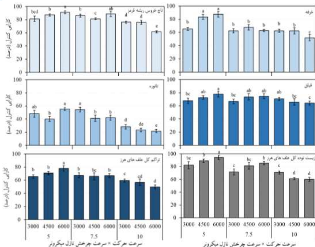
شکل ۵. اثر سرعت حرکت و سرعت چرخش نازل میکروتر پهیپاد مدل EFT-G620 بر تراکم و وزن علف‌های هرز. میانگین‌ها با حرف مشترک براساس آزمون چند دامنه‌ای دانکن در سطح احتمال ۵ درصد تفاوتی ندارند.
