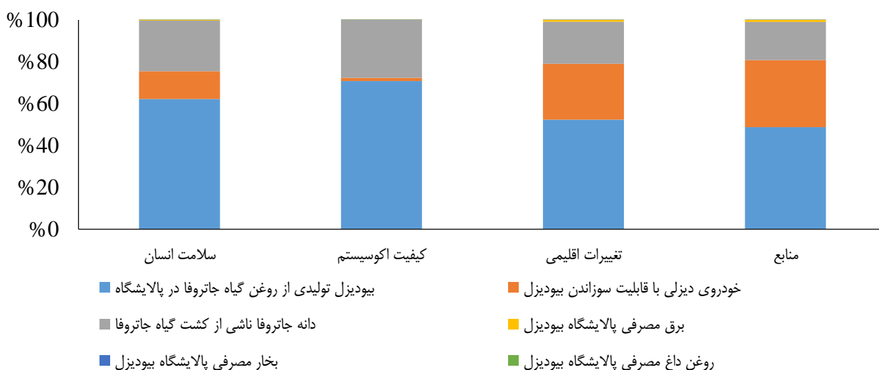
شکل ۵. سهم هریک از بخش‌های تولید در صدمات زیست‌محیطی چرخه حیات خودروی بیودیزلی
