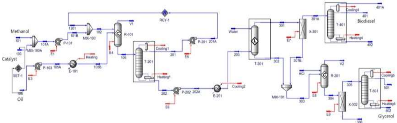
شکل ۳. شبیه‌سازی فرآیند واحد تولید بیودیزل از روغن گیاه جاتروفا در نرم‌افزار هایسیس (منبع: یافته‌های تحقیق)
