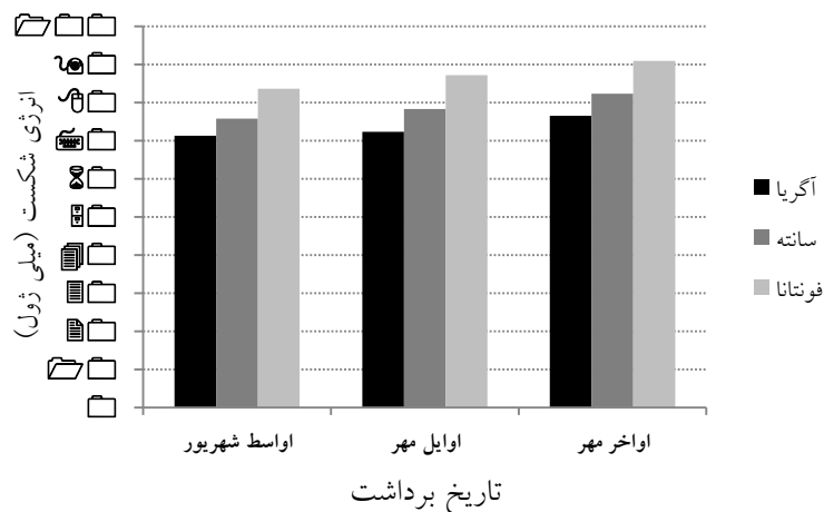
شکل ۵. تأثیر تاریخ برداشت و رقم بر میزان انرژی شکست سبب زمینی
