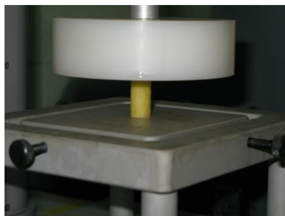
شکل ۲- نمونه سیب زمینی مورد استفاده در آزمایش فشار
