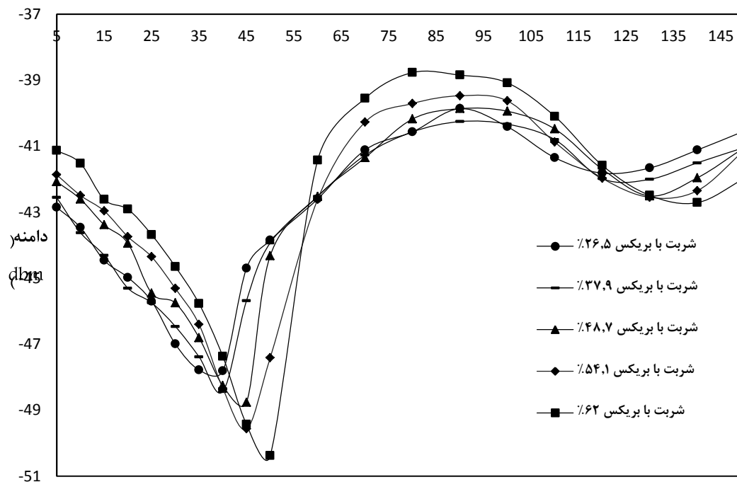
شکل ۵. طیف‌های دامنه-فرکانس (A-F) شربت چغندر قند در غلظت‌های مختلف
