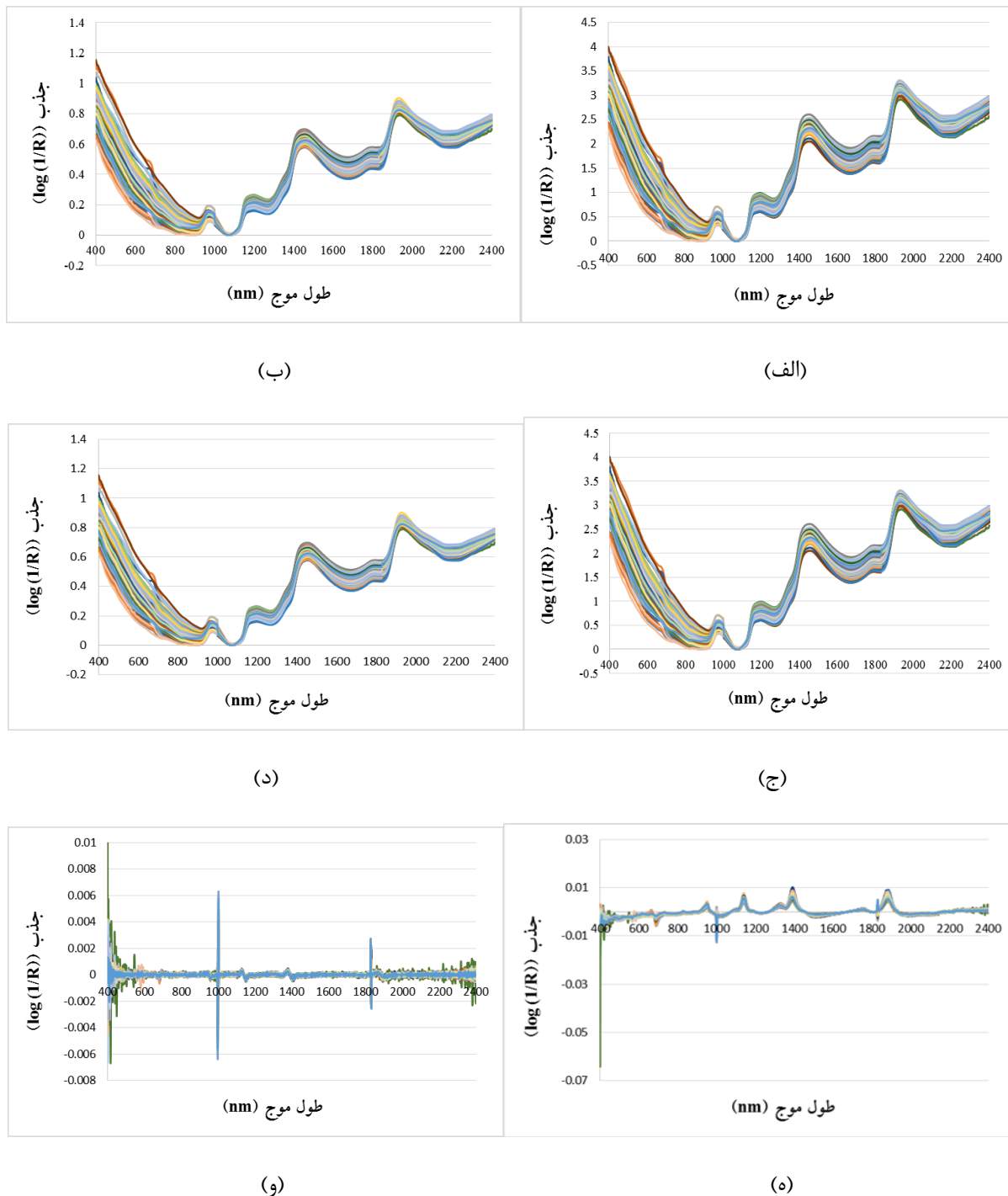
شکل ۴. طیف‌های جذبی NIR نمونه‌های چغندر قند پردازش شده با ترکیب روش‌های (الف) MA+SNV، (ب) MA+MSC، (ج) SG+SNV، (د) SG+MSC، (ه) SG+D1، (و) SG+D2
