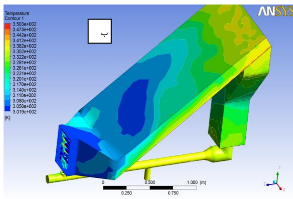
شکل ۸. توزیع کانتورهای دما در ساعت ۱۲:۰۰ به وقت محلی با دبی ۰/۰۰۶ کیلوگرم بر ثانیه برای خروجی اول برای الف) صفحه گذرنده از مرکز سامانه، ب) دیواره خارجی سیال جاری در جمع کننده، خشک کن و مبدل حرارتی.
