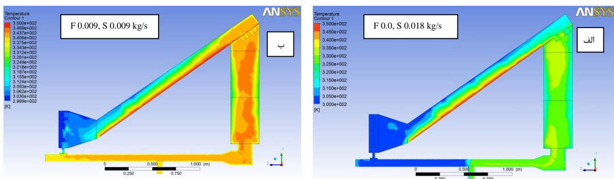
شکل ۷. توزیع کانتورهای دما در ساعت ۱۲:۰۰ به وقت محلی برای دبی های متفاوت برای خروجی اول و خروجی دوم
