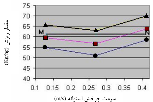
شکل ۵- میزان ریزش برای سطوح مختلف سرعت در مقایسه با شاهد تعداد انگشتی: ۱۸ ● تعداد انگشتی: ۱۴ ■ تعداد انگشتی: ۱۰ ▲
