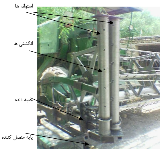
شکل ۱- قطعات عمده و چگونگی نصب دستگاه جدا کننده بر روی پلاتفرم کمباین
