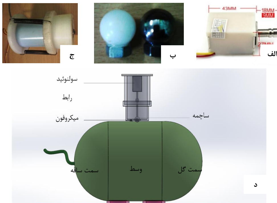
شکل ۲. نمایی از اجزای سیستم اخذ سیگنال صوتی: الف) سولنوئید ب) ساچمه‌ها ج) محفظه سیستم ضربه‌زن د) شماتیک کلی و موقعیت‌های اعمال ضربه و اخذ سیگنال آکوستیک
