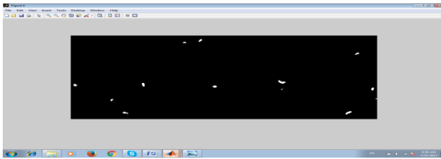
شکل ۹. تصویر باینری
