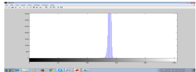
شکل ۱۰. هیستوگرام تصویر
