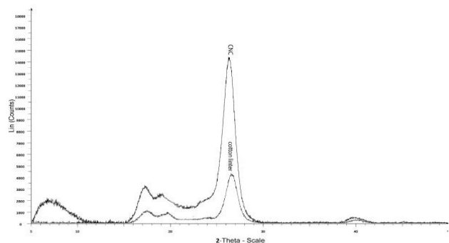
شکل ۵. نمودار پراش پرتو ایکس سلولز و نانو کریستال سلولز (طیف بالایی مربوط به نانوکریستال سلولز و طیف پایینی مربوط به الیاف پنبه می باشد).
