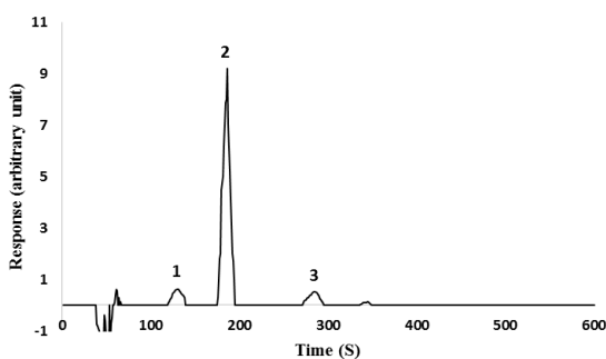
شکل ۱. نمودار مربوط به آزمون HPLC نمونه استخراج شده
